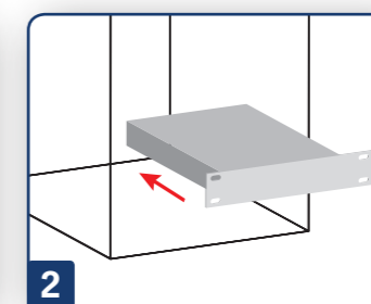
Einbau Seite links und rechts
